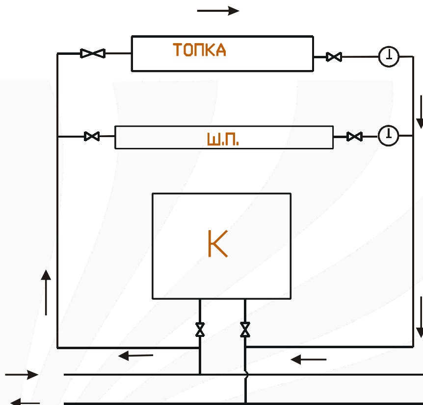
Рис.3 Схема охлаждения топки с шурующей планкой.
