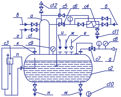
Принципиальная схема подключения деаэратора
