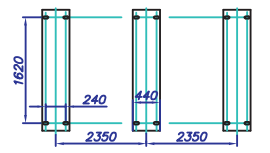
Схема расположения отверстий в опорах
