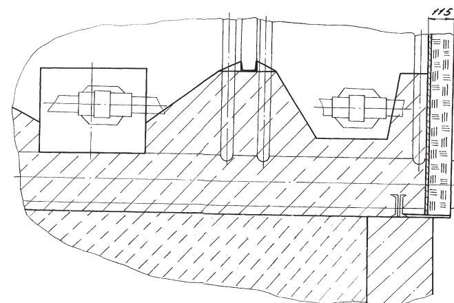
И-И (1:10) (4)
