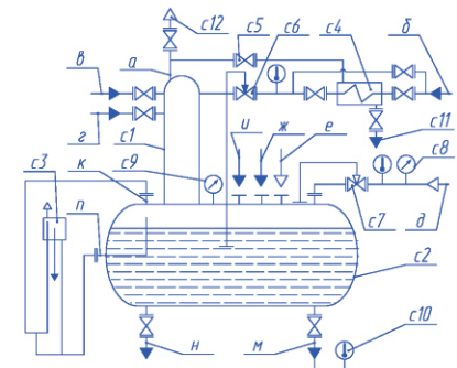
Принципиальная схема подключения деаэратора ДА 100/25
